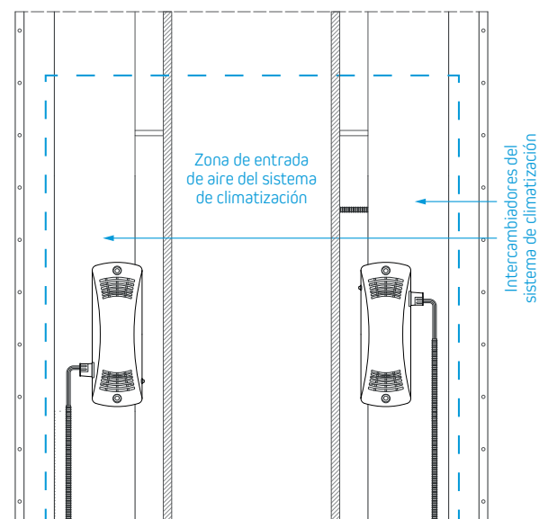
Vista inferior: Una zona de entrada de aire de los sistemas de climatización dentro del vehículo.
